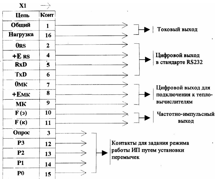
X1 - вилка 2РМТ24КПН19Ш1В1В ГЕО.364.126 ТУ Рисунок В.1 - Кабель «ВЫХОД»
