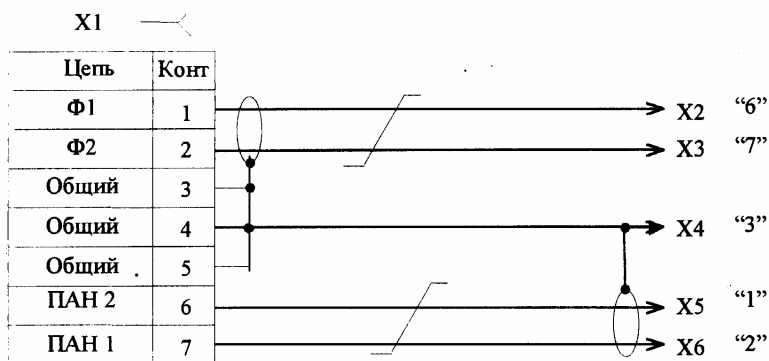
X1 - вилка 2РМТ18КПН7Ш1В1В ГЕО.364.126 ТУ X2 - X6 - наконечники 1-47-25 ОСТ 1 13704-81 Рисунок В.2 - Кабель «ППР7-ИП7»
