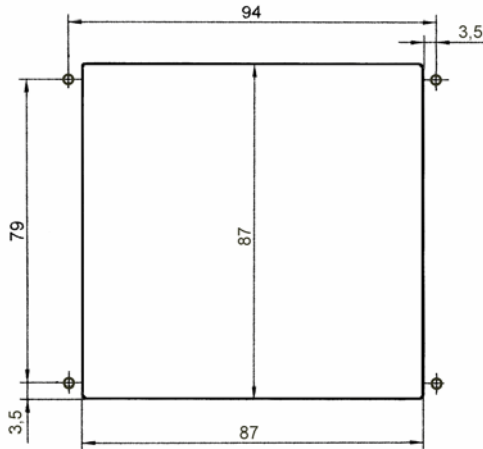
Рис. 2. Габариты окна и разметка отверстий для установки индикатора на щите
