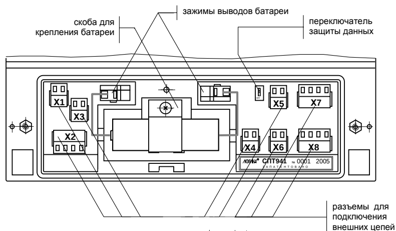
Рисунок 3.2 – Монтажный отсек тепловычислителя СПТ941.11
