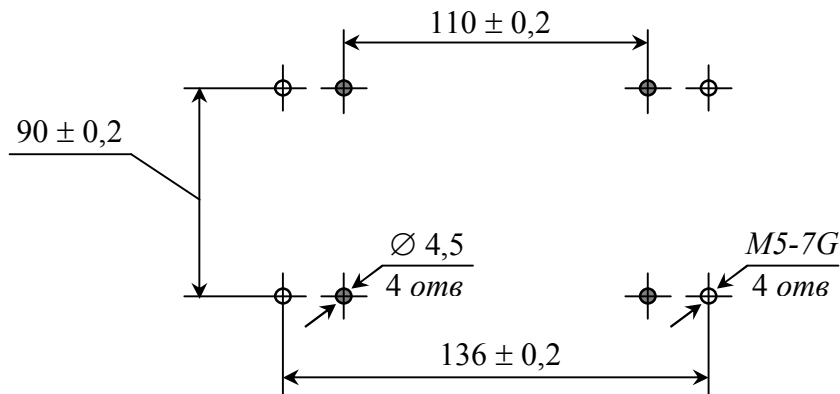
Рисунок 2 – Разметка для крепления ВТД-В
